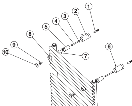
Σχήμα 5: Εξαρτήματα συναρμολόγησης
