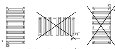
Σχήμα 8: Σωστή τοποθέτηση
