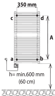
Figura 6: Dimensiuni montaj a,b,c,d suporturi montaj
