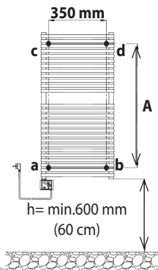
Slika 6: Oznake za rupe
