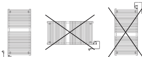
Abbildung 8: Richtige und falsche Anwendungsarten des Handtuchheizkörpers.
