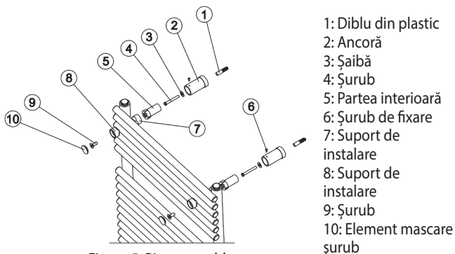
Figura 5: Piese asamblare
